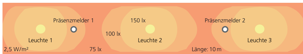
Grundriss eines Korridors mit Leuchten und Isolux-Kurven
