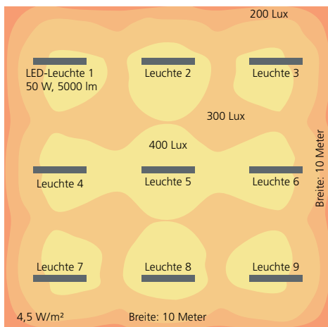
Grundriss einer Werkstatt mit Leuchten und Isolux-Kurven
