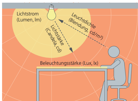
Zusammenhang zwischen der Beleuchtungsstärke und den Leuchten- und Lampenkennwerten Lumen und Candela sowie der Blendung
